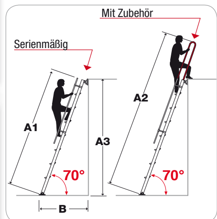
Obere gerade Handläufe (Best.-Nr. S15-MCVER)
