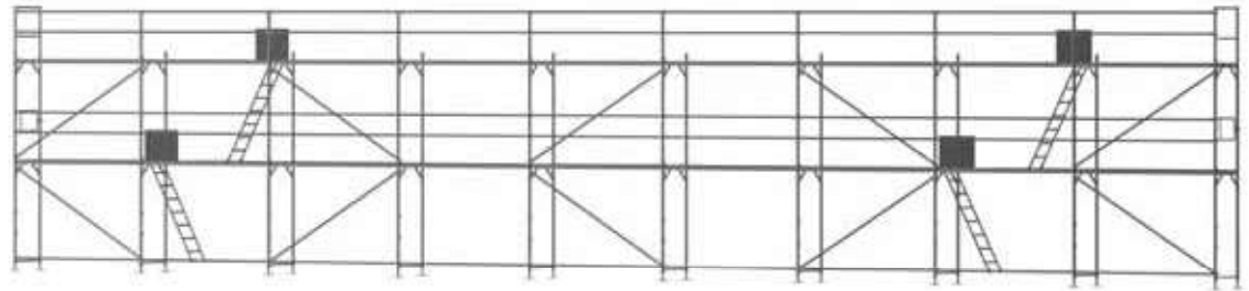
Variante 1: Giebelgerüst
