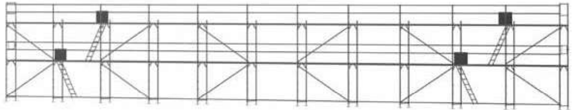
Variante 1: Giebelgerüst
