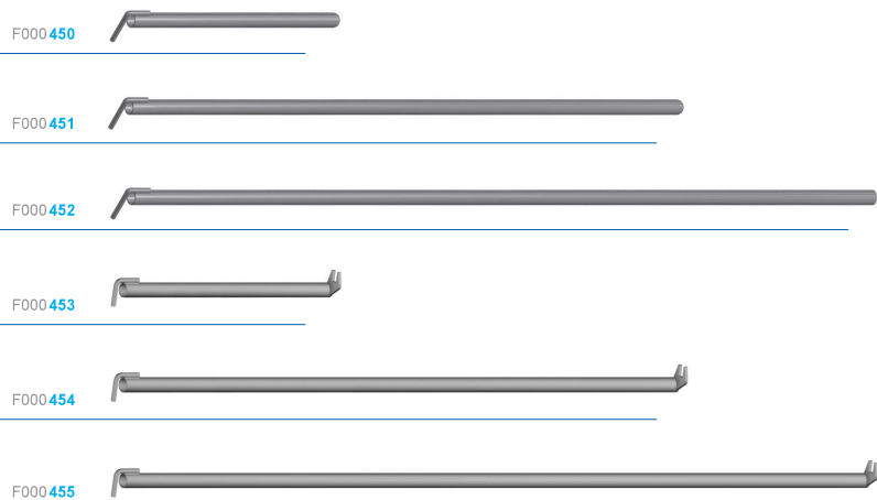
F000456 L = 0,50m F000457 L = 1,50m F000458 L = 2,00m Gerüstankerrohr Doppelkupplung starr Ringschraube 100 mm Spreizdübel Abdeckkappe
