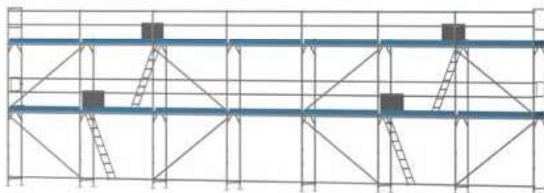
Variante 1: Giebelgerüst
