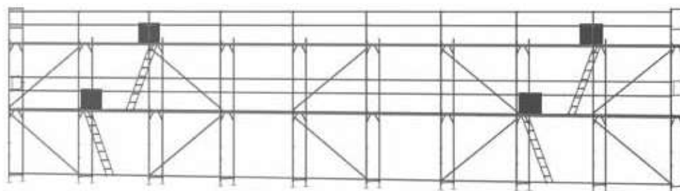
Variante 1: Giebelgerüst
