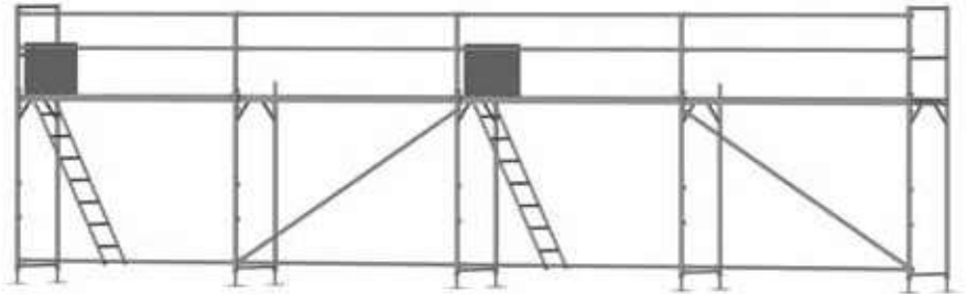
Variante 1: Giebelgerüst
