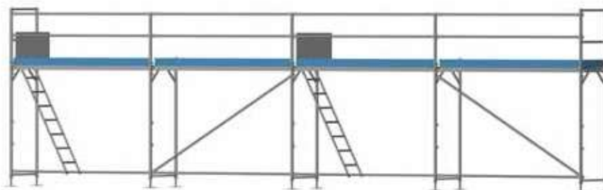
Variante 1: Giebelgerüst
