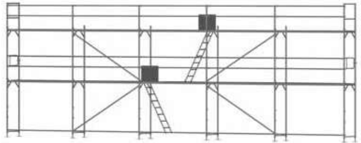
Variante 1: Giebelgerüst
