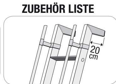
Geschweißte Wandabstandshalter (Best.-Nr. S15/D15).
