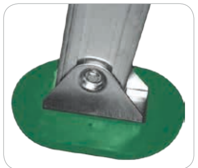
ZUBEHÖR: 16x11 cm ovaler schwenkbarer Gelenkfuß. Die Struktur aus Stahl mit Gummi verhindert, dass der Fuß in den Boden einsinkt.
