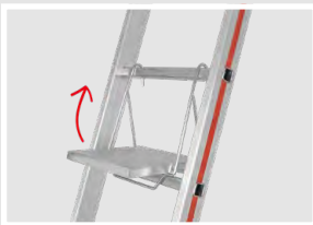
Einhängetritt für Sprossenleitern Siehe Seite 90 ▪ Best.-Nr. 0050378 260×250 mm, klappbar ▪ Best.-Nr. 005411 300×255 mm
