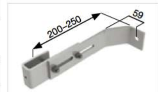
Abb. Bestell-Nr. 60022, 62022, 64022
