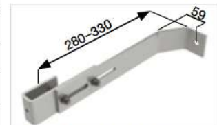
Abb. Bestell-Nr. 60023, 62023, 64023
