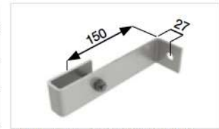
Abb. Bestell-Nr. 60018, 62018, 64018
